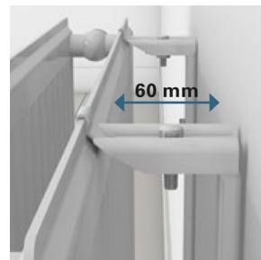
Alltid 60 mm mellan radiator och vägg ger god åtkomst för rengöring.
